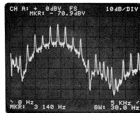
modem
